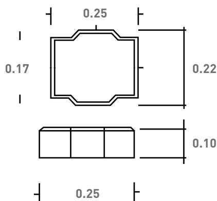
ADOQUÍN 22X25X10CM
